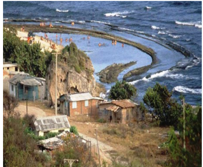
FIGURA 1. Aspectos más frecuentes de las rocas de playa: izquierda. Frente a la desembocadura del río Yacabo Abajo, sureste provincia Guantánamo: de estratos gruesos y levantadas sobre el nivel medio del mar. Derecha. Ensenada en la desembocadura del río San Juan (playa Agüadores), sur de la Sierra Maestra: de estratos finos, con su superficie al nivel medio del mar, semejando pliegues, debido a que adoptan la morfología del lugar, constituidas. Constituidas en ambos casos, principalmente, por litoclastos.
